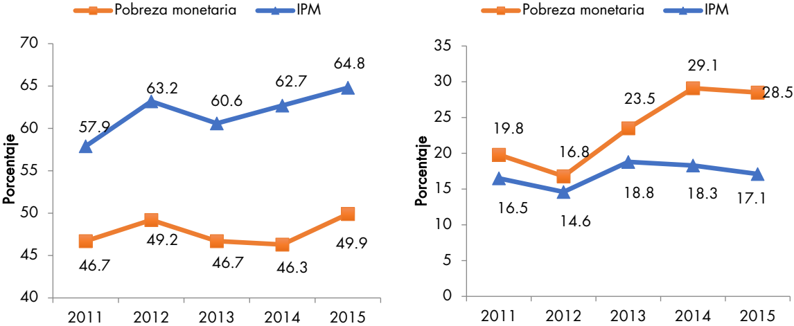
Gráfico 3. Errores de inclusión y exclusión para puntajes inferiores a 50 Panel A. Errores de inclusión Panel B. Errores de exclusión
